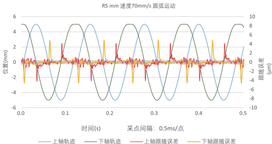
半径5mm圆, 加工速度70mm/s, 动态跟随误差10μm (下轴SMH225LM, 上轴SMH190LM)
